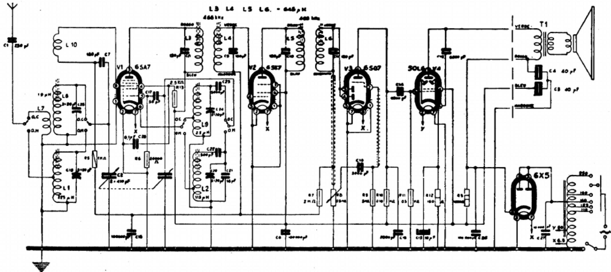
DUCATI RR 2051 - Schema Elettrico.
